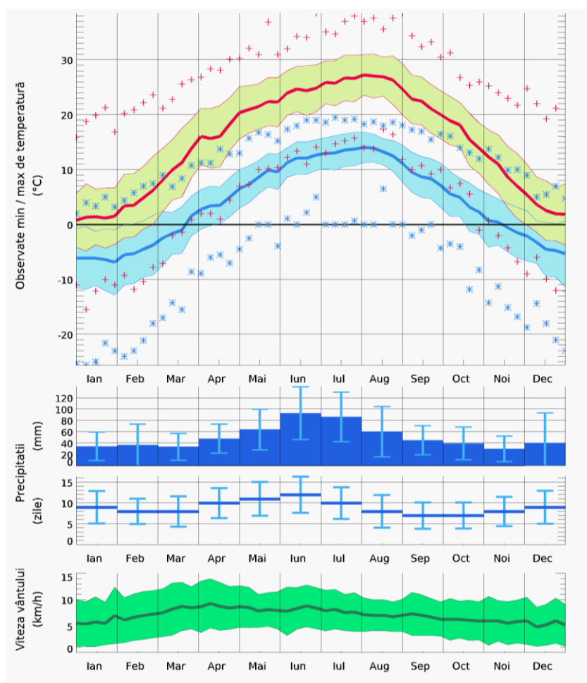
Tendențe meteorologice locale în Municipiul Cluj-Napoca
