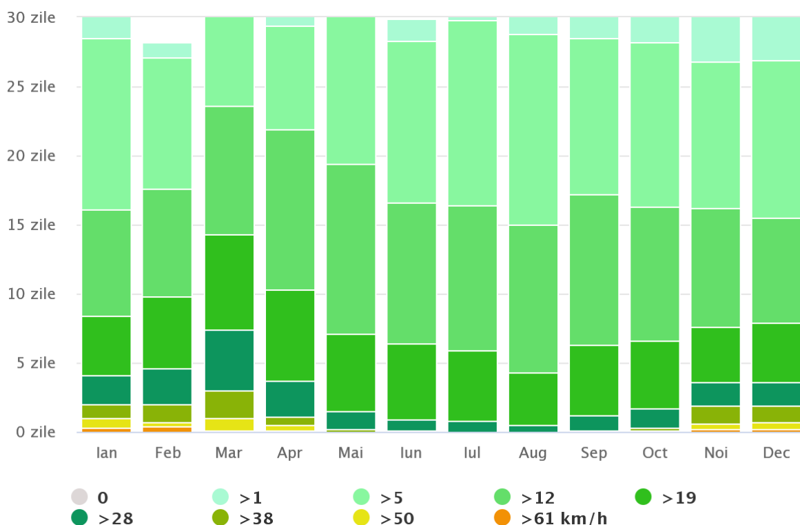
Mișcarea maselor de aer
